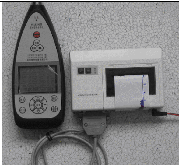
图 10-7 数据打印
