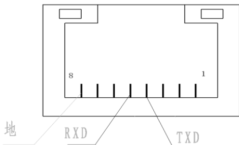
图 3-5 RS 232 接口
